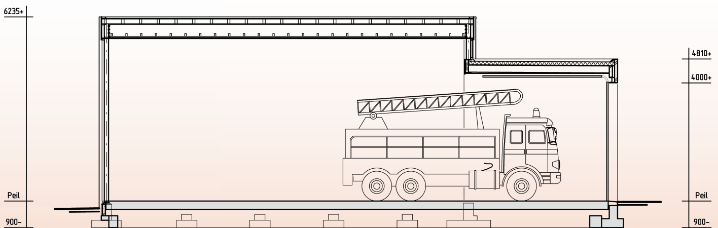
Dwarsdoorsnede nieuwe situatie
